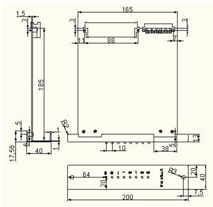
圖 3-8 燈號驅動模組尺寸
