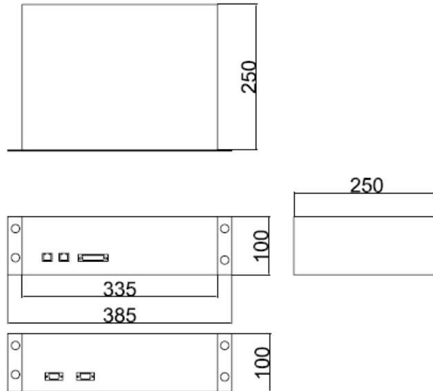
圖 3-7 通訊監控模組尺寸
