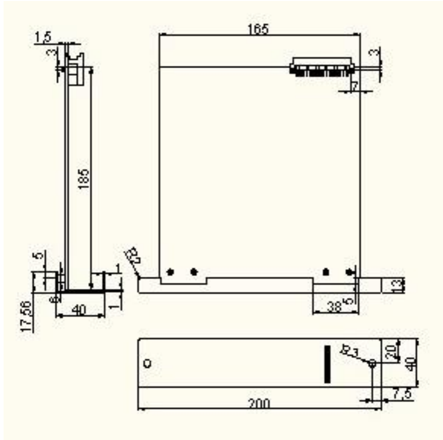
圖 3-9 號誌備援模組尺寸
