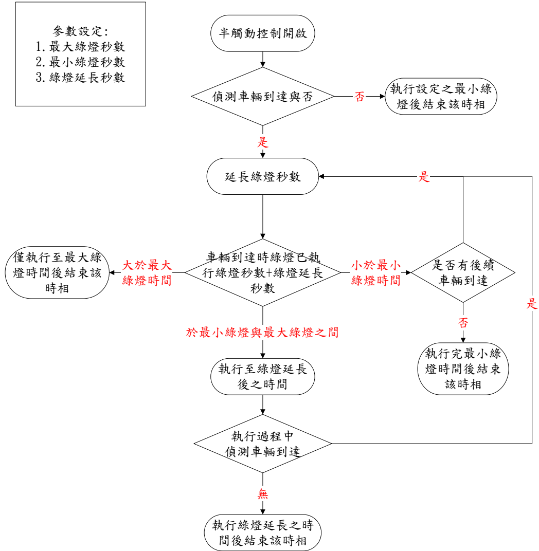
圖 5-1 全(半)觸動號誌控制流程
